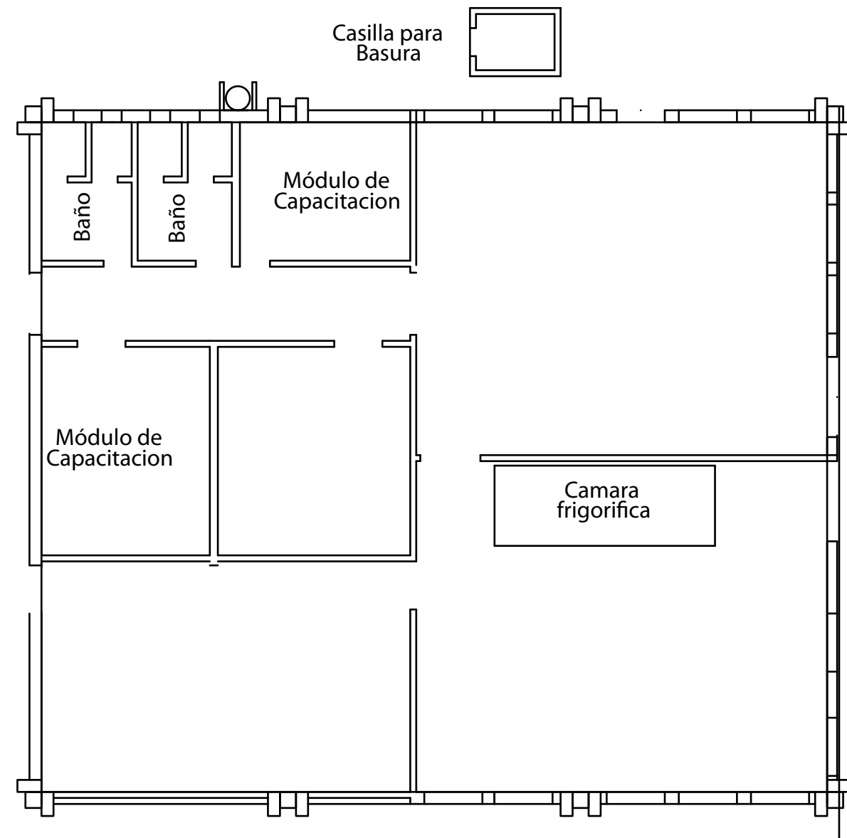
Planta Baja
